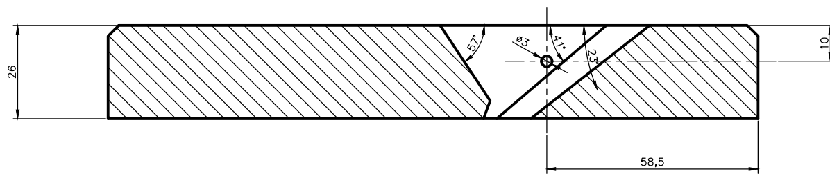
COUPE A-A
